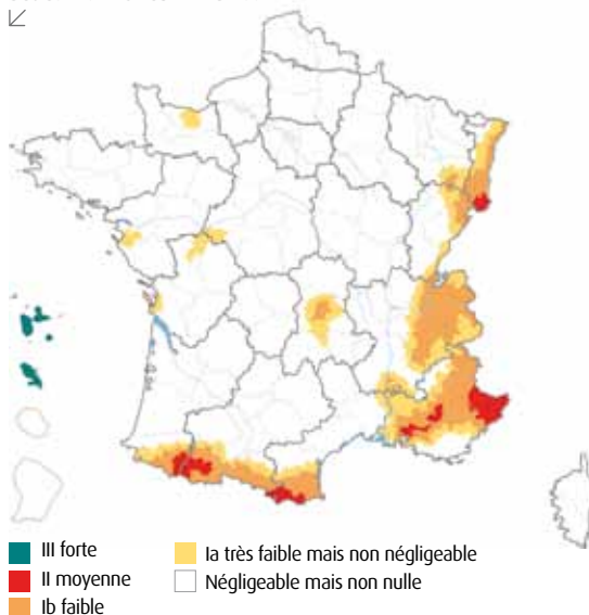
Ancien zonage sismique (jusqu'au 30/04/2011) Décret n° 91-461 du 11 mai 1991
