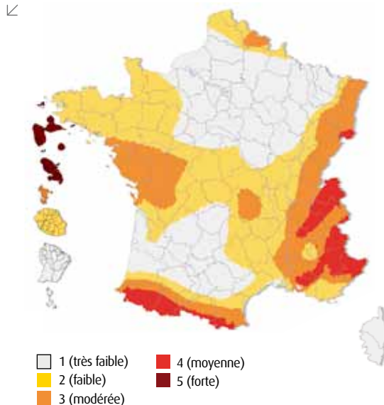
Nouveau zonage sismique (depuis le 01/05/2011) Décret n° 2010-1255 du 22 octobre 2010
