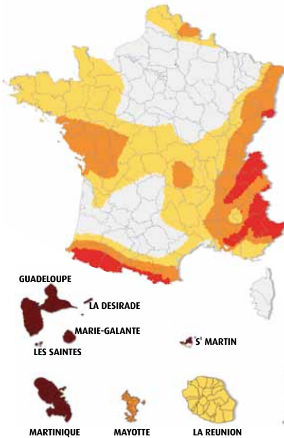
▮ Zonage sismique de la France en vigueur depuis le 1 er mai 2011 (décret n o 2010-1255)
